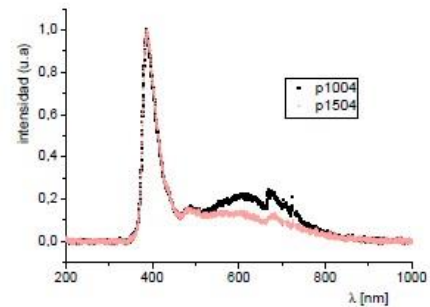
Figura 5: Espectro de fotoluminiscencia de las muestras P1004 y P1504.
